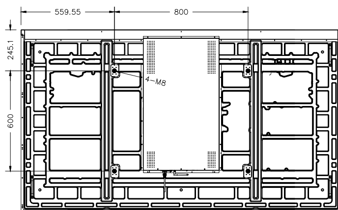
СХЕМА ДИСПЛЕЯ (ВИД СЛЕВА)
