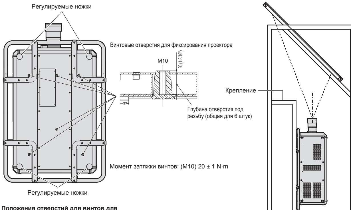
Положения отверстий для винтов для фиксирования проектора и регулируемых ножек
