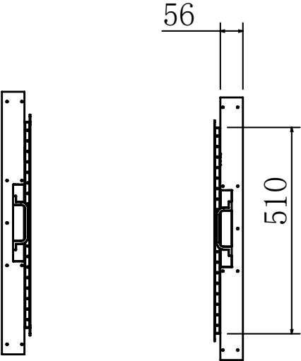
СХЕМА ДИСПЛЕЯ (ВИД СПРАВА И СЛЕВА)
