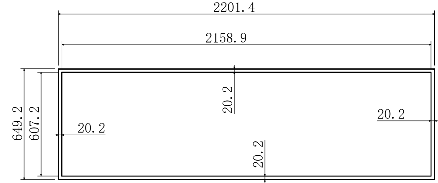
СХЕМА ДИСПЛЕЯ (ВИД СПЕРЕДИ)
