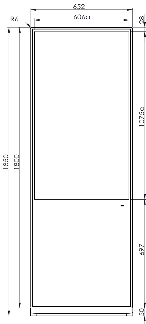
СХЕМА ДИСПЛЕЯ (ВИД СПЕРЕДИ)
