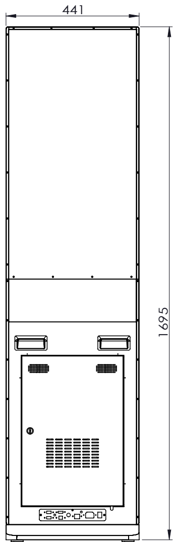
СХЕМА ДИСПЛЕЯ (ВИД СЗАДИ)
