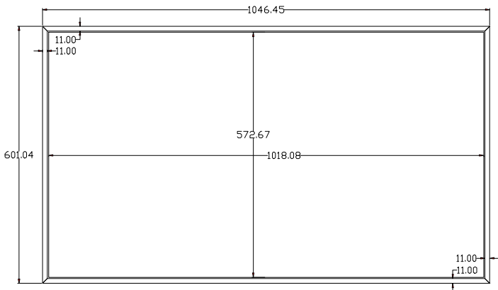
СХЕМА ДИСПЛЕЯ (ВИД СПЕРЕДИ)
