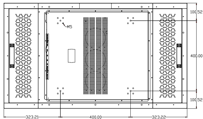
СХЕМА ДИСПЛЕЯ (ВИД СЗАДИ)
