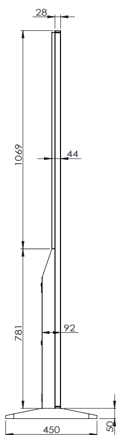
СХЕМА ДИСПЛЕЯ (ВИД СЛЕВА)
