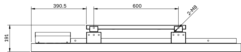
СХЕМА ДИСПЛЕЯ (ВИД СНИЗУ)
