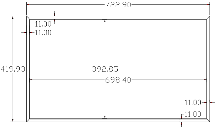
СХЕМА ДИСПЛЕЯ (ВИД СПЕРЕДИ)
