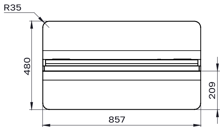
СХЕМА ДИСПЛЕЯ (ВИД СВЕРХУ)
