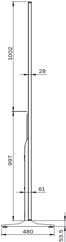
СХЕМА ДИСПЛЕЯ (ВИД СЛЕВА)
