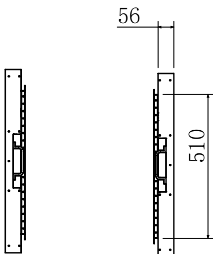
СХЕМА ДИСПЛЕЯ (ВИД СПРАВА И СЛЕВА)
