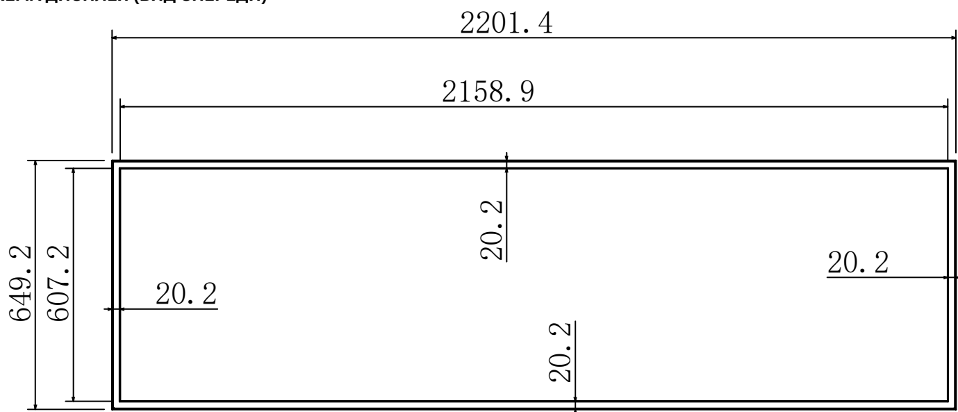
СХЕМА ДИСПЛЕЯ (ВИД СПЕРЕДИ)
