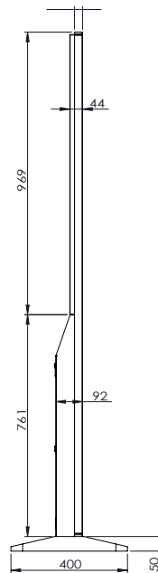
СХЕМА ДИСПЛЕЯ (ВИД СЛЕВА)
