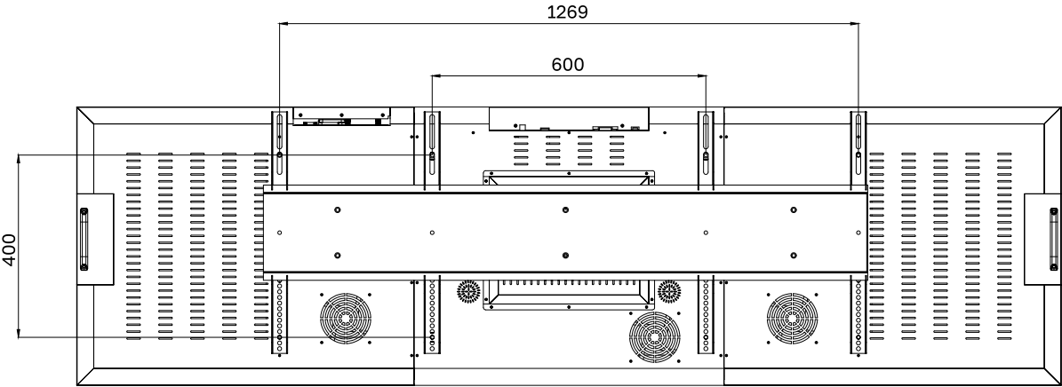
СХЕМА ДИСПЛЕЯ (ВИД СЗАДИ)
