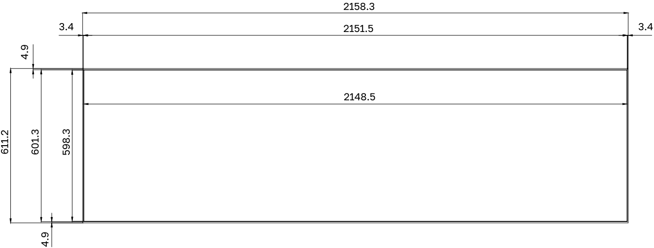
СХЕМА ДИСПЛЕЯ (ВИД СЗАДИ)
