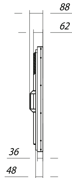
СХЕМАТИЧНОЕ ИЗОБРАЖЕНИЕ (ВИД СБОКУ)
