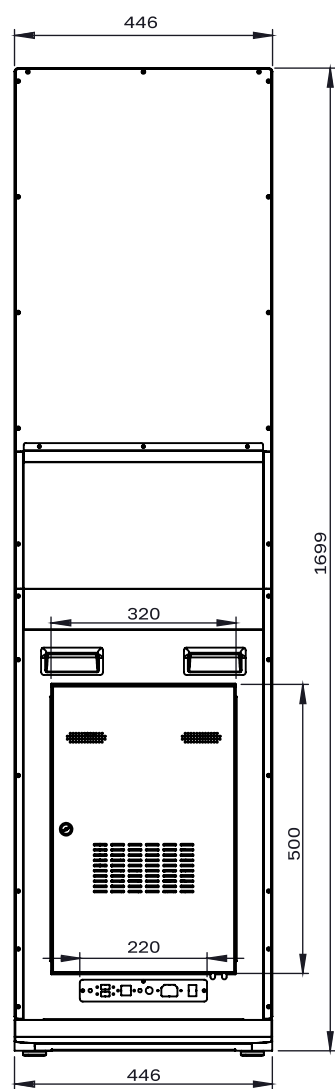
СХЕМА ДИСПЛЕЯ (ВИД СЗАДИ)
