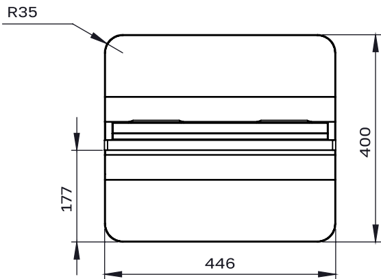
СХЕМА ДИСПЛЕЯ (ВИД СВЕРХУ)
