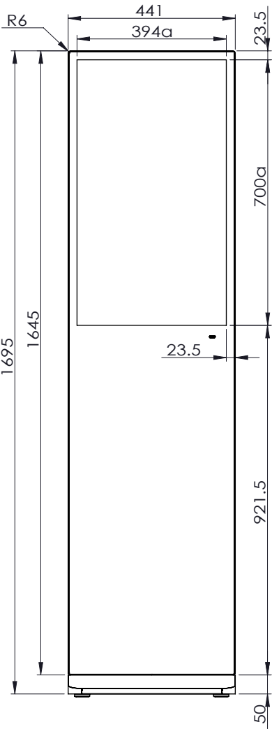
СХЕМА ДИСПЛЕЯ (ВИД СПЕРЕДИ)
