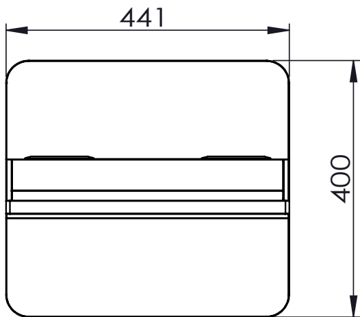
СХЕМА ДИСПЛЕЯ (ВИД СВЕРХУ)
