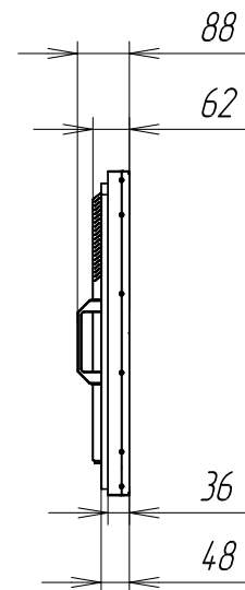
СХЕМАТИЧНОЕ ИЗОБРАЖЕНИЕ (ВИД СБОКУ)
