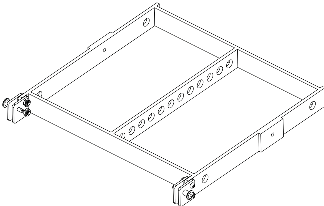
Рама для подвеса (1 шт.)
