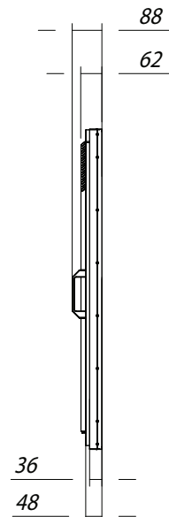
СХЕМАТИЧНОЕ ИЗОБРАЖЕНИЕ (ВИД СБОКУ)
