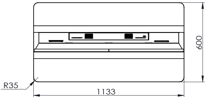
СХЕМА ДИСПЛЕЯ (ВИД СВЕРХУ)
