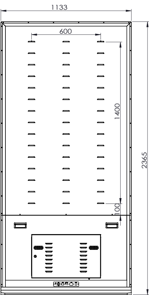
СХЕМА ДИСПЛЕЯ (ВИД СЗАДИ)
