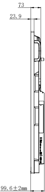
СХЕМА ПАНЕЛИ (ВИД СЛЕВА)
