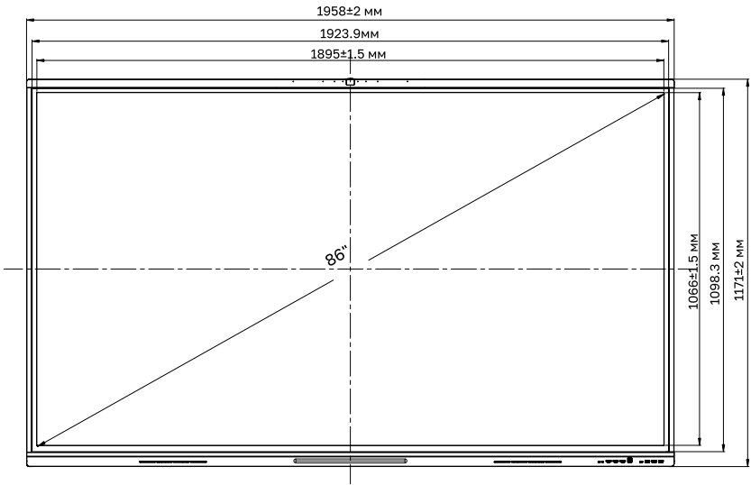
СХЕМА ПАНЕЛИ (ВИД СПЕРЕДИ)
