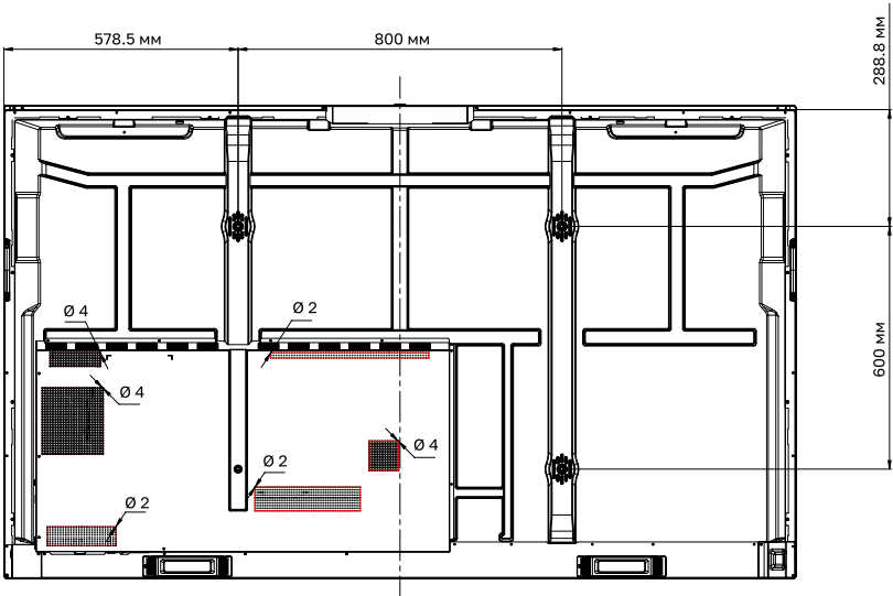
СХЕМА ПАНЕЛИ (ВИД СЗАДИ)
