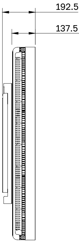
СХЕМА ДИСПЛЕЯ (ВИД СЛЕВА)
