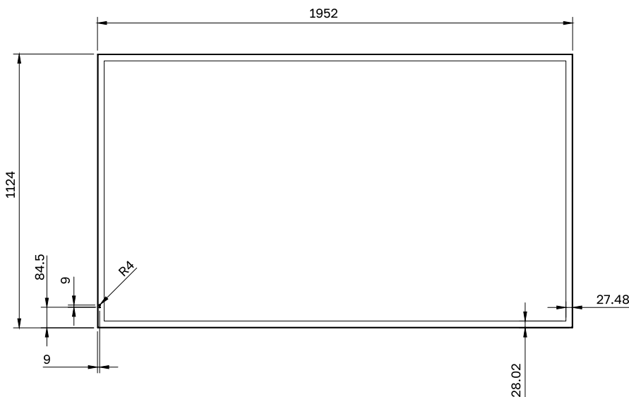
СХЕМА ДИСПЛЕЯ (ВИД СПЕРЕДИ)
